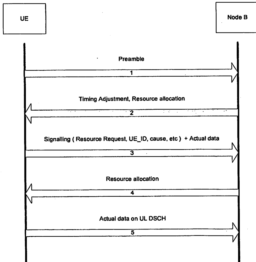
[도 5]. 상향 링크 동기가 유지하지 않을 때 자원 할당 방법
