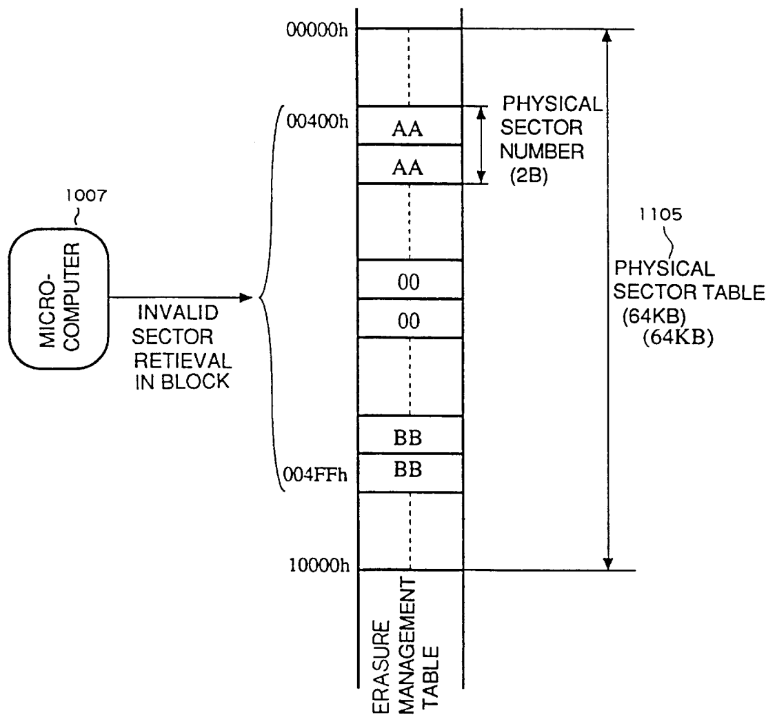
FIG. 27 PSRAM
