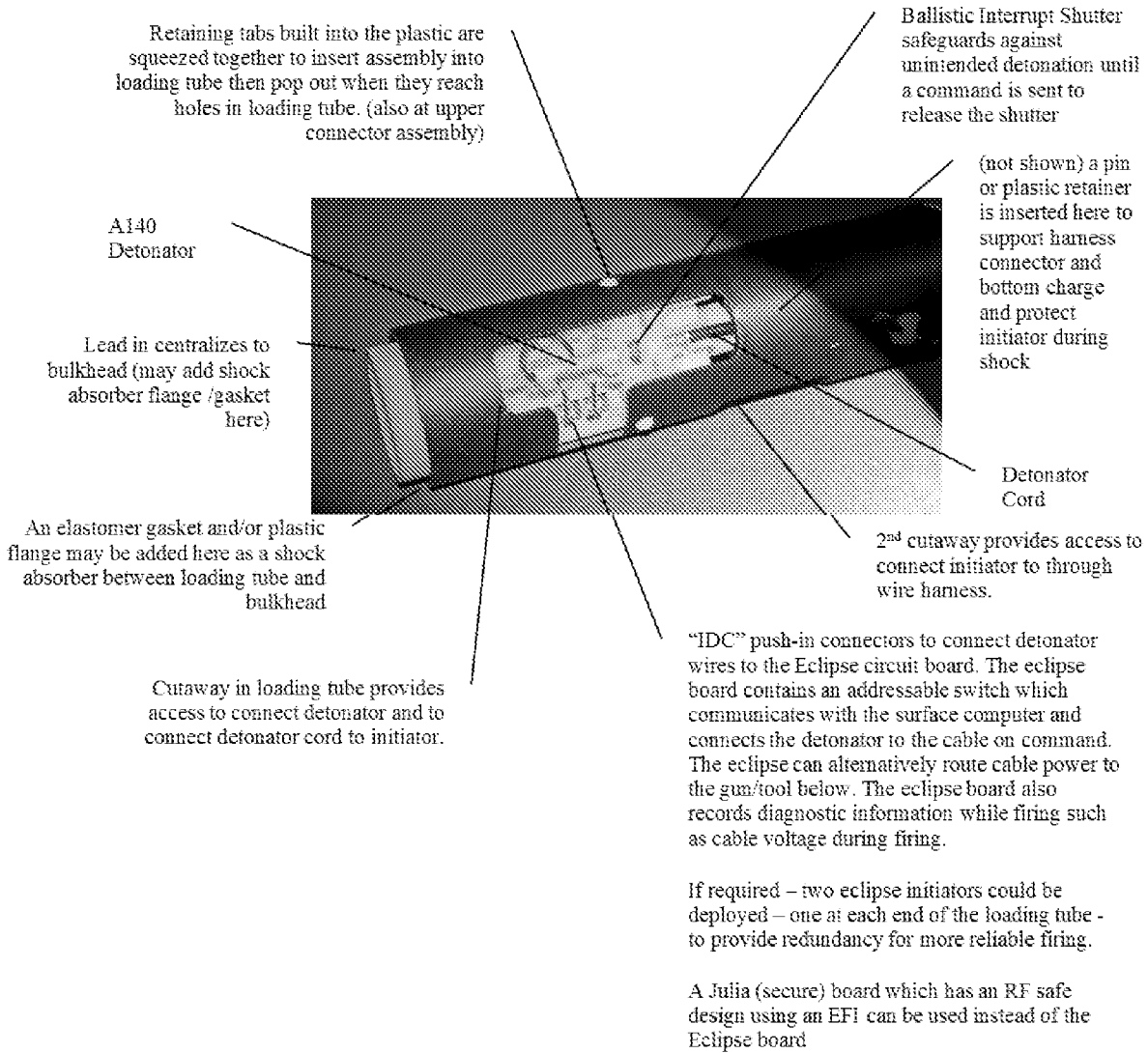
Fig. 4: Eclipse initiator
