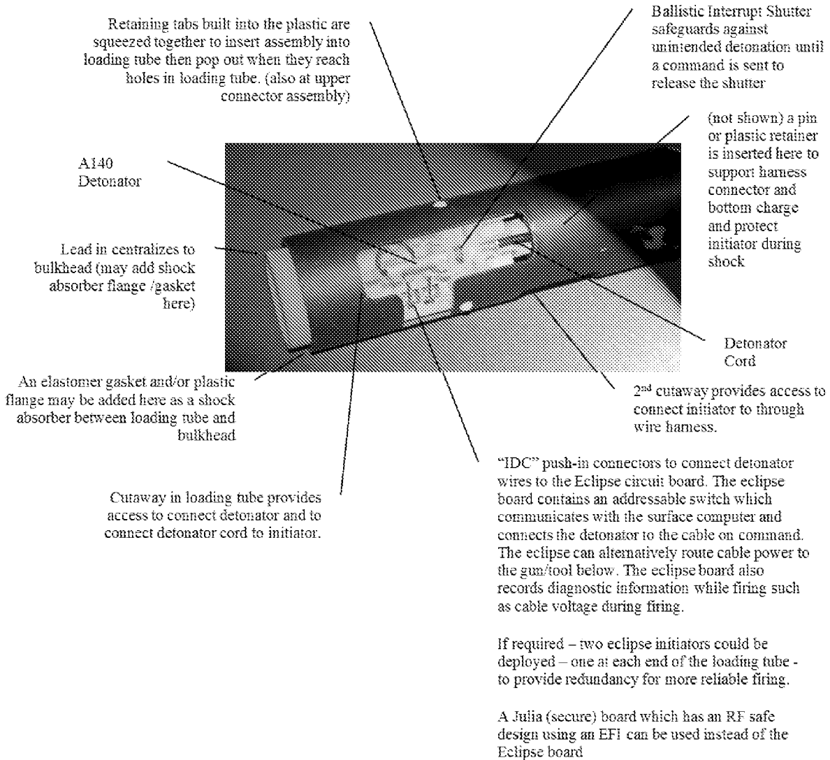
Fig. 4: Eclipse initiator
